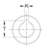
Keyway
